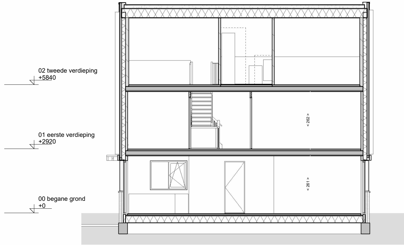
dwarsdoorsnede
