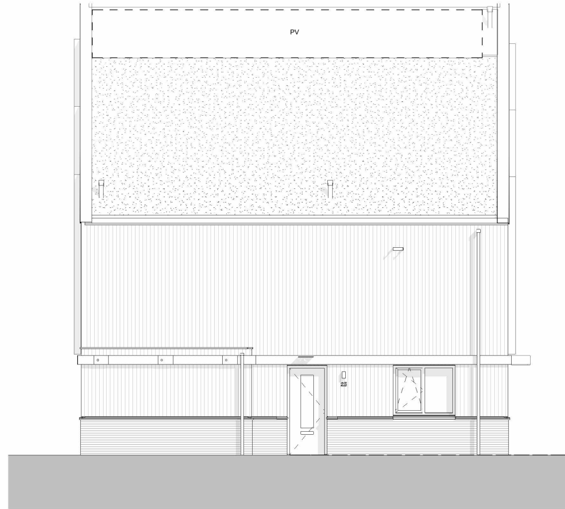
zijgevel (noordwest)
